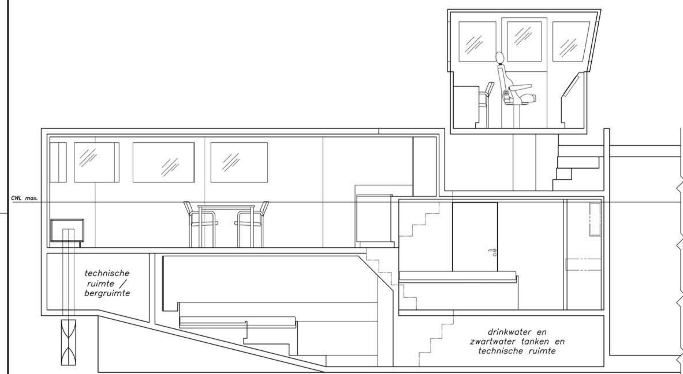
langsdoorsnede
