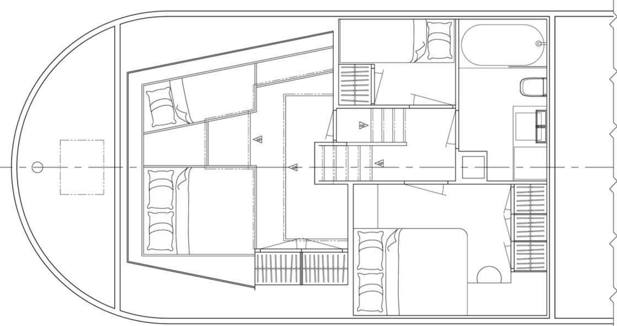
bovenaanzicht slaapkamers en badkamer
