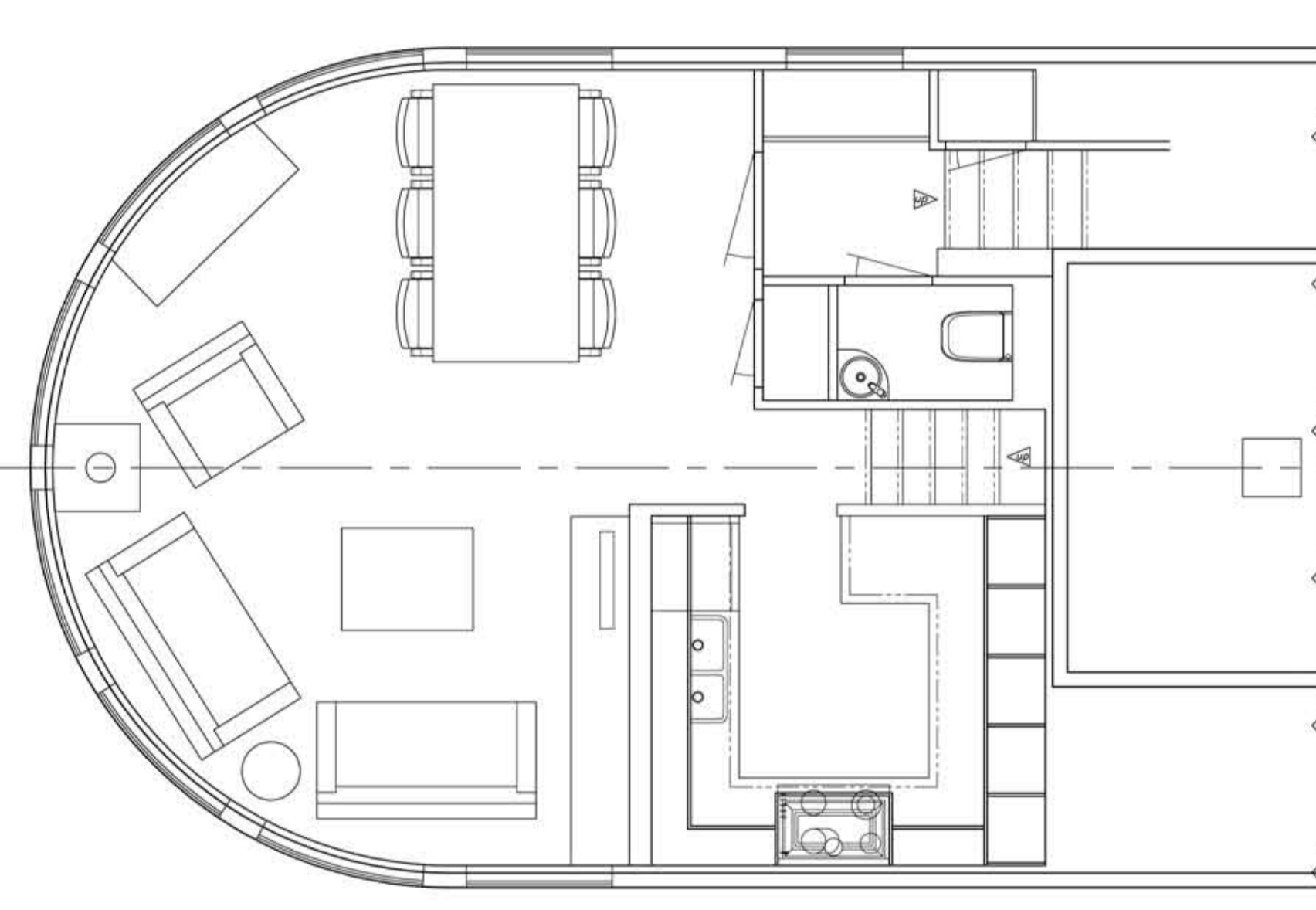
bovenaanzicht woonruimte
